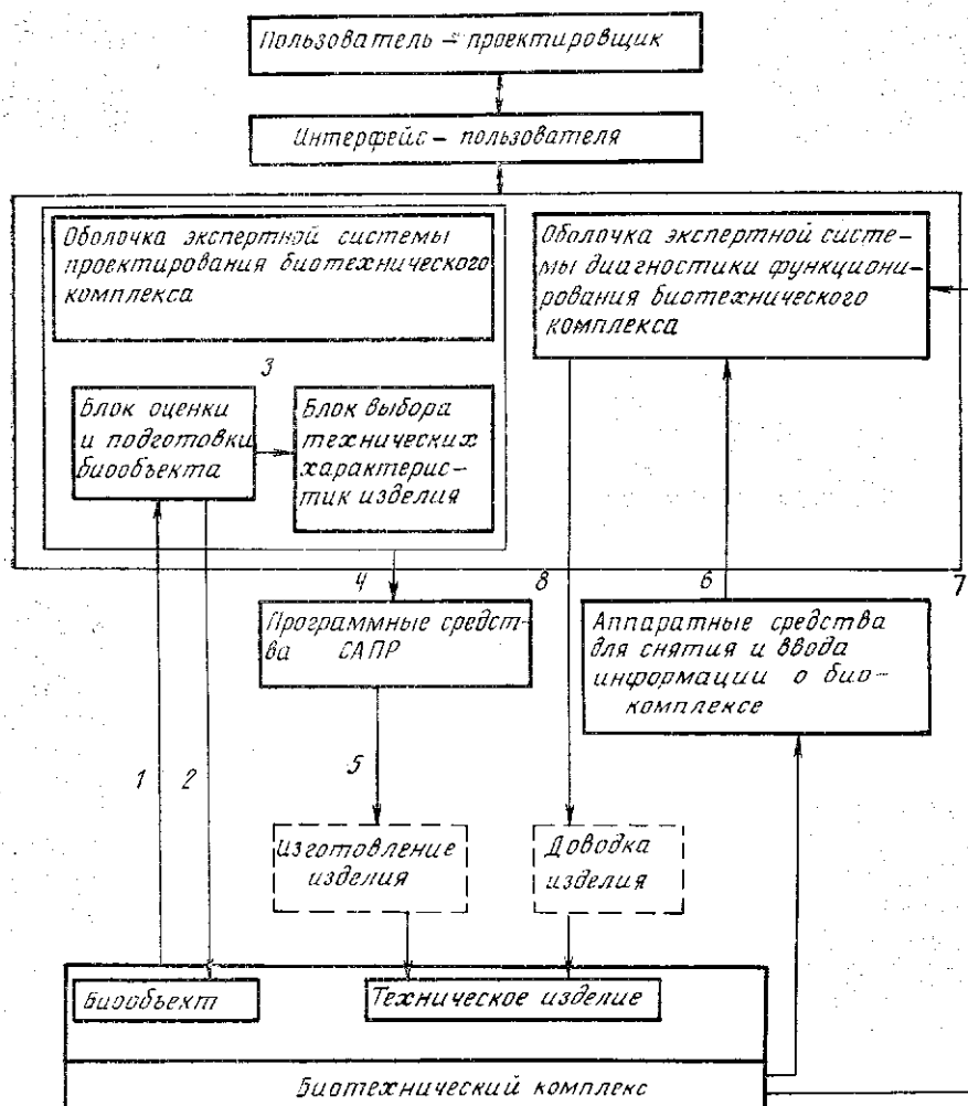
Рис. 1. Архитектура гибридной экспертной системы проектирования и диагностики биотехнических изделий. 1 - Индивидуальные характеристики биообъекта, 2 - Рекомендации по подготовке биообъекта к функционированию в составе биокомплекса, 3 - Функциональные требования, предъявляемые к техническому изделию, 4 - Технические характеристики изделия, 5 - Управляющая программа для станка с ЧПУ, 6 - Данные объективного исследования функционирования биокомплекса, 7 - Данные визуального наблюдения за функционированием биокомплекса, 8 - Рекомендации по доводке изделия
